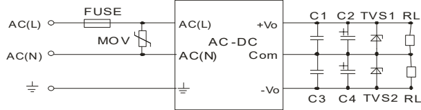
图2: 正负双路典型应用电路
