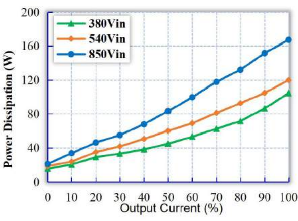
图(2):Tcase=25℃,分别在最小输入电压,额定输入电压,最大输入电压时,不同负载时的损耗.
