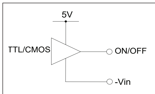
图 F: TTL/CMOS 控制方式
