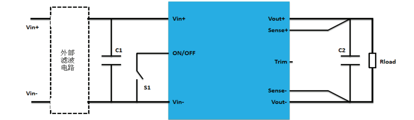
图 A: 典型应用电路
