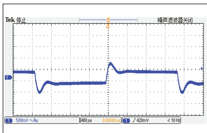
图 3: 输出纹波电压, Vin=280V, Io=17.9A, TC=25°C
