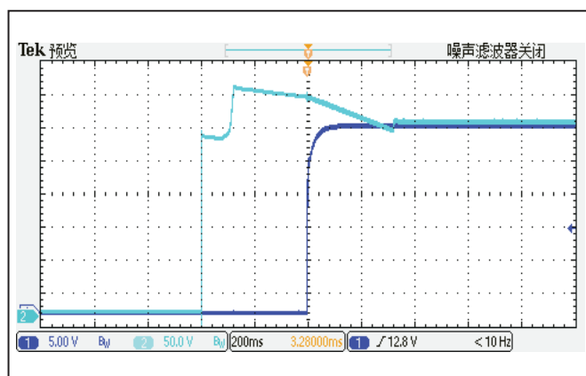
图 5: 启机延时, Vin=280V, Io=17.9A, TC=25°C CH1: 输出电压, CH2: 输入电压
