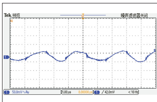
图 4: 负载动态响应, Vin=280V, Io=17.9A, Io=50%-75%-50%, 2.5A/µs, TC=25°C, CH1: 输出电压
